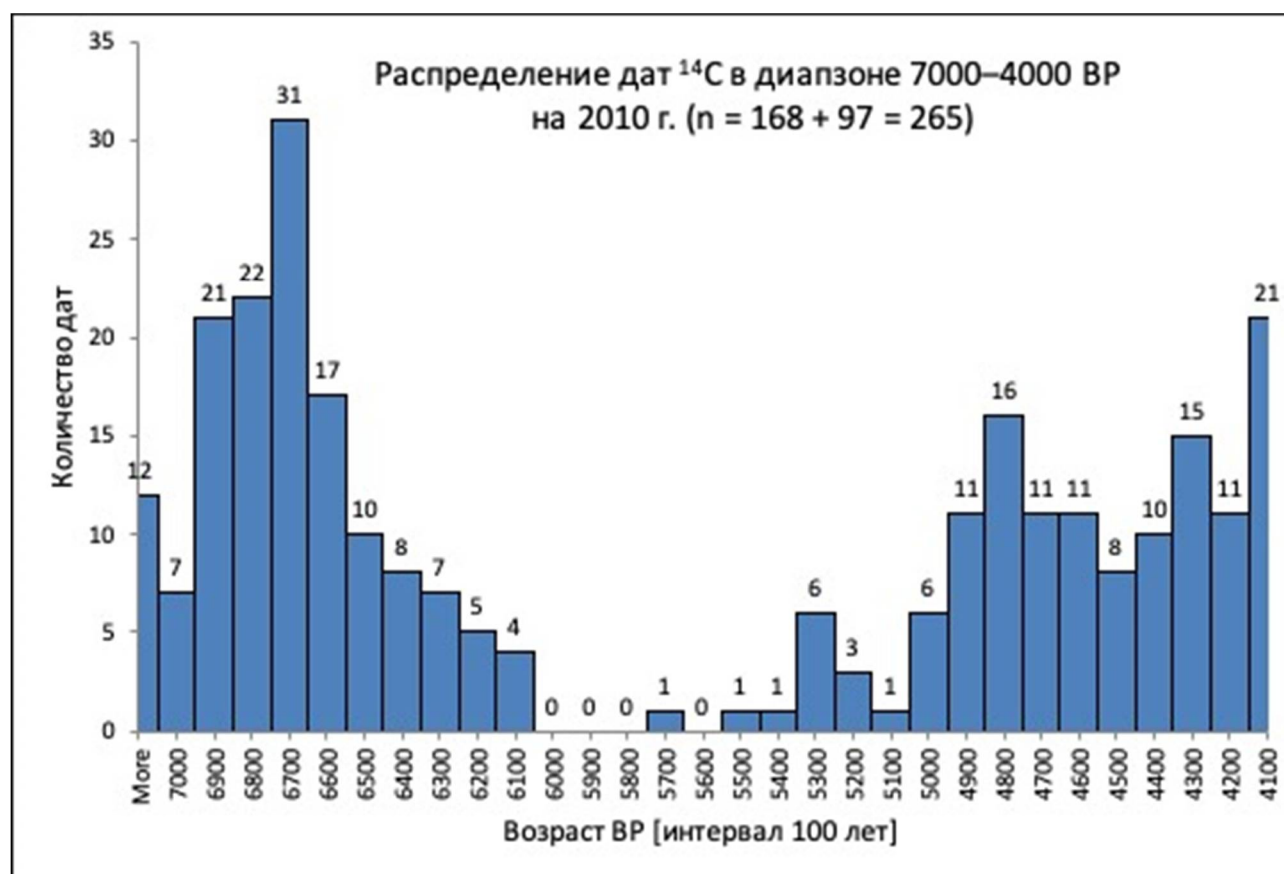
Рис. 3. Распределение AMS и сцинтилляционных дат ^{14}\text{C} в диапазоне 7000–4000 ВР для человеческих костяков позднего мезолита – позднего неолита в Предбайкалье на 2010 г. (Мамонова, Сулержицкий, 1989; Weber et al., 2006; Weber, McKenzie, Beukens, 2010)
